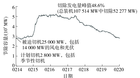
图4 发电机组停机容量变化
