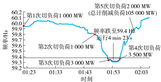
图3 2021年2月15日凌晨得州电网频率变化曲线
