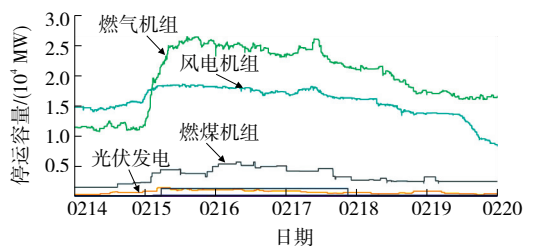
图5 不同类型发电机组停机容量
