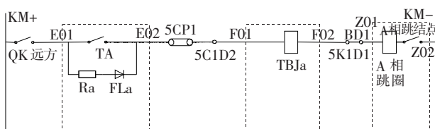
图 7 一条完整的控制回路原理示意
