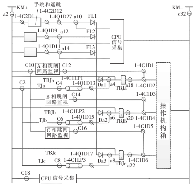
图 11 跳闸回路跳闸状态
