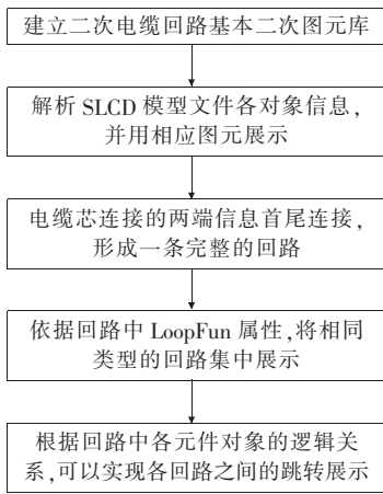
图 5 二次电缆回路可视化流程
