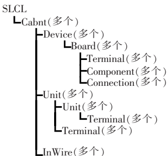
图 3 CLCD 文件模型结构
