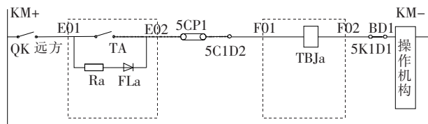
图 6 屏柜中的某一条控制回路
