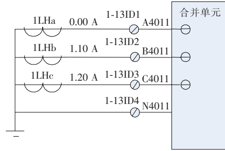
图 9 测量回路在线监测示意
