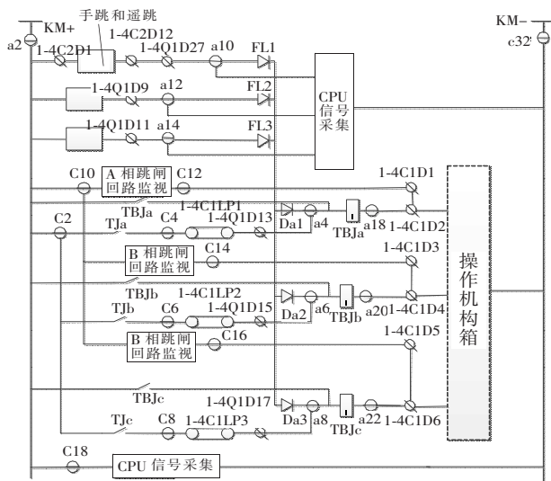
图 10 智能终端跳闸回路
