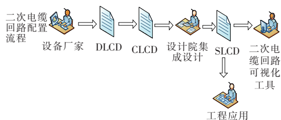
图1 二次电缆回路设计流程
