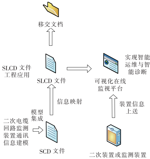
图 8 工程化应用流程
