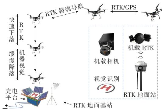
图 1 系统结构流程
