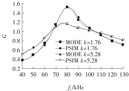
图 8 PSIM 和运行模态分析法电压增益曲线对比
