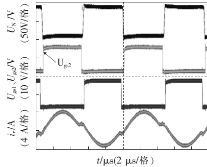
(b) 基于模态分析的样机运行波形
