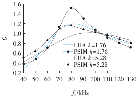
图 7 PSIM,FHA 电压增益曲线对比
